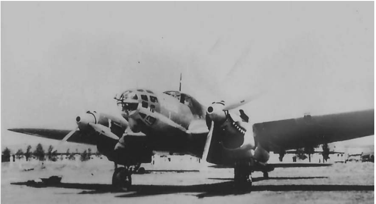
“Pedro 1” 25-3 mostrando las tomas de aire suplementarias de sus motores, el montaje de la ametralladora de proa semicircular y la cubierta de la ventilación del carburador larga, características de los Heinkel He.111 B-0.
