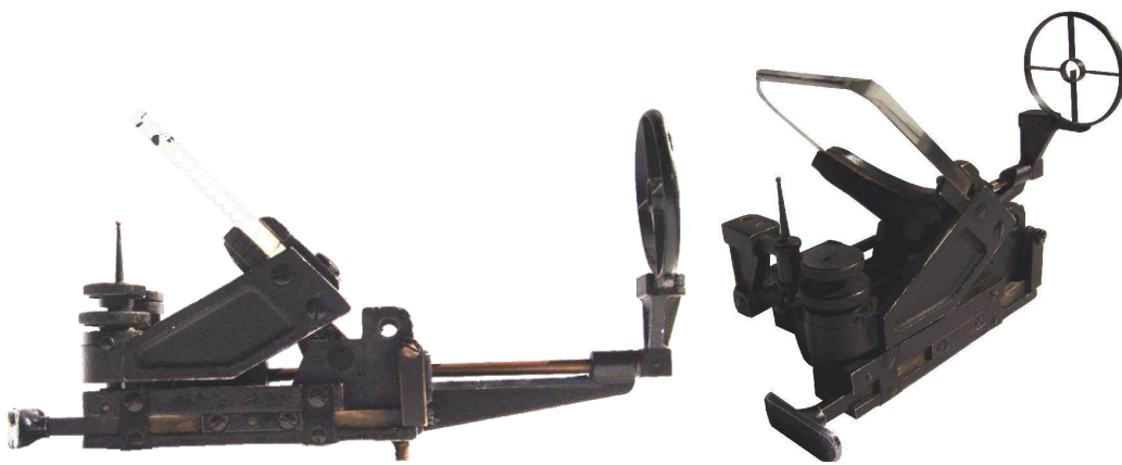
Imágenes de detalle del Reflexvisier 3a.
