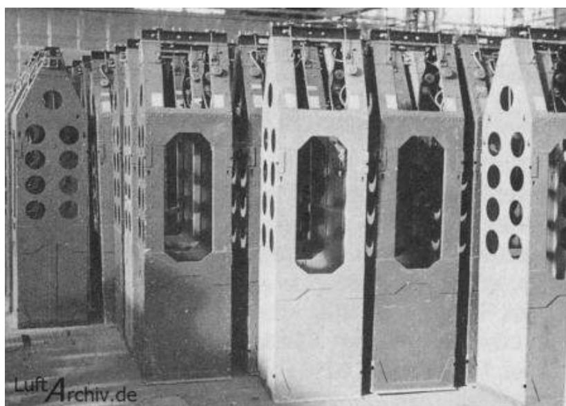
Lanzabombas ESAC/250/IX usados por los Heinkel He.111, individualizados, como puede verse.
