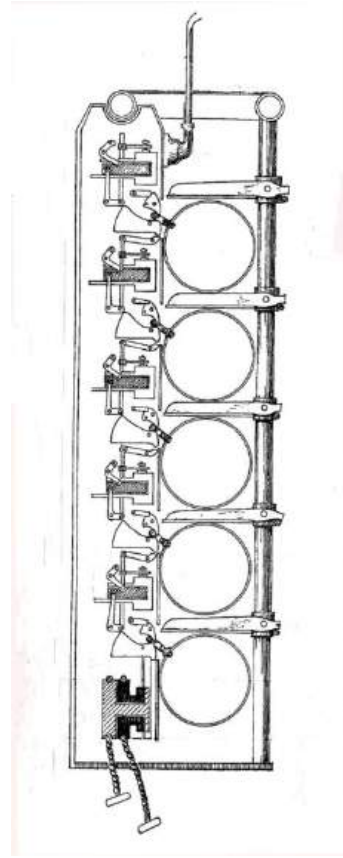
Lanzabombas horizontal Maga 5. C-50 y su corte esquemático frontal. El Do.17 E llevaba uno a cada lado de la bahía de bombas. Como bombardero no era una gran cosa.
