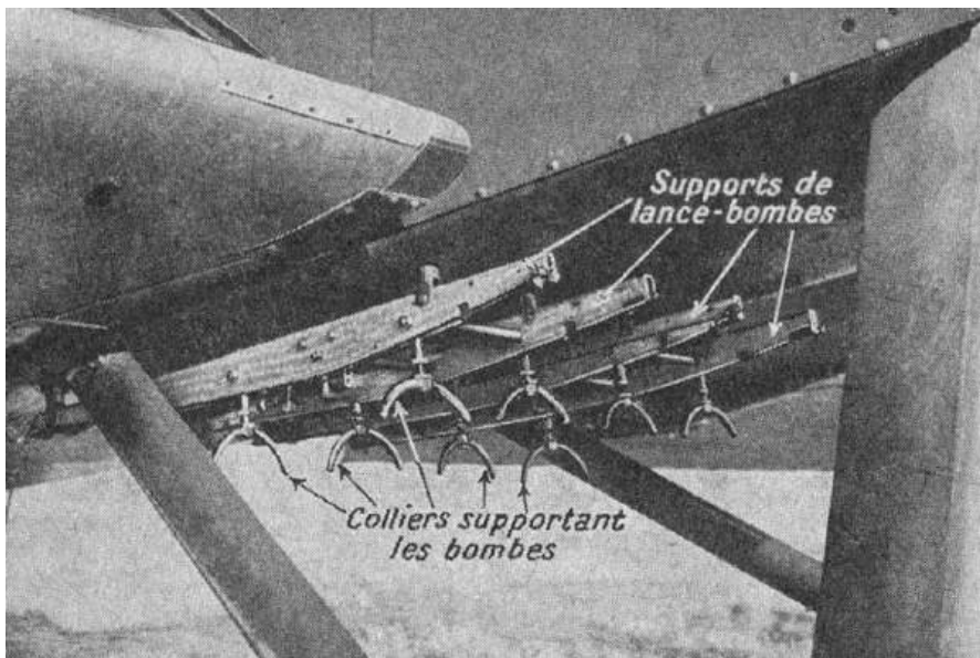
Lanza-bombas ventral de un Potez 25 para cuatro bombas de 50 kilogramos.
