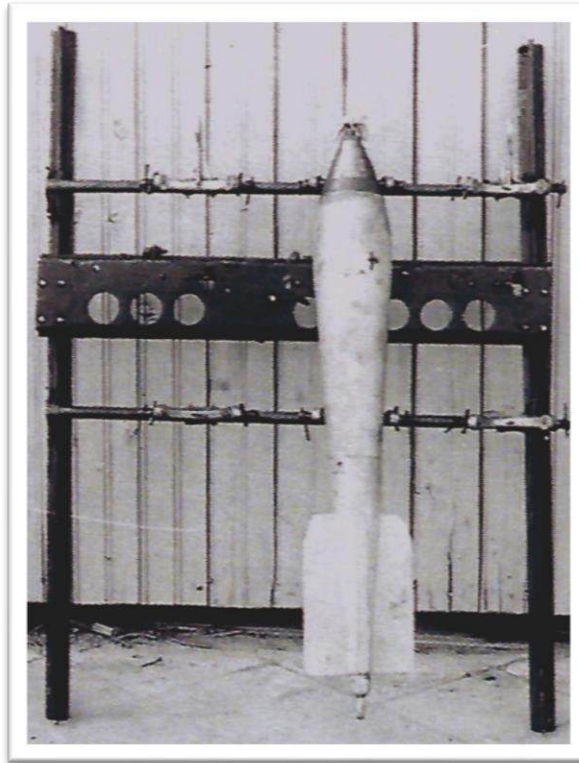
Bomba “Hispania” Mod. A.5 presentada en un lanzabombas horizontal 3-A-5
