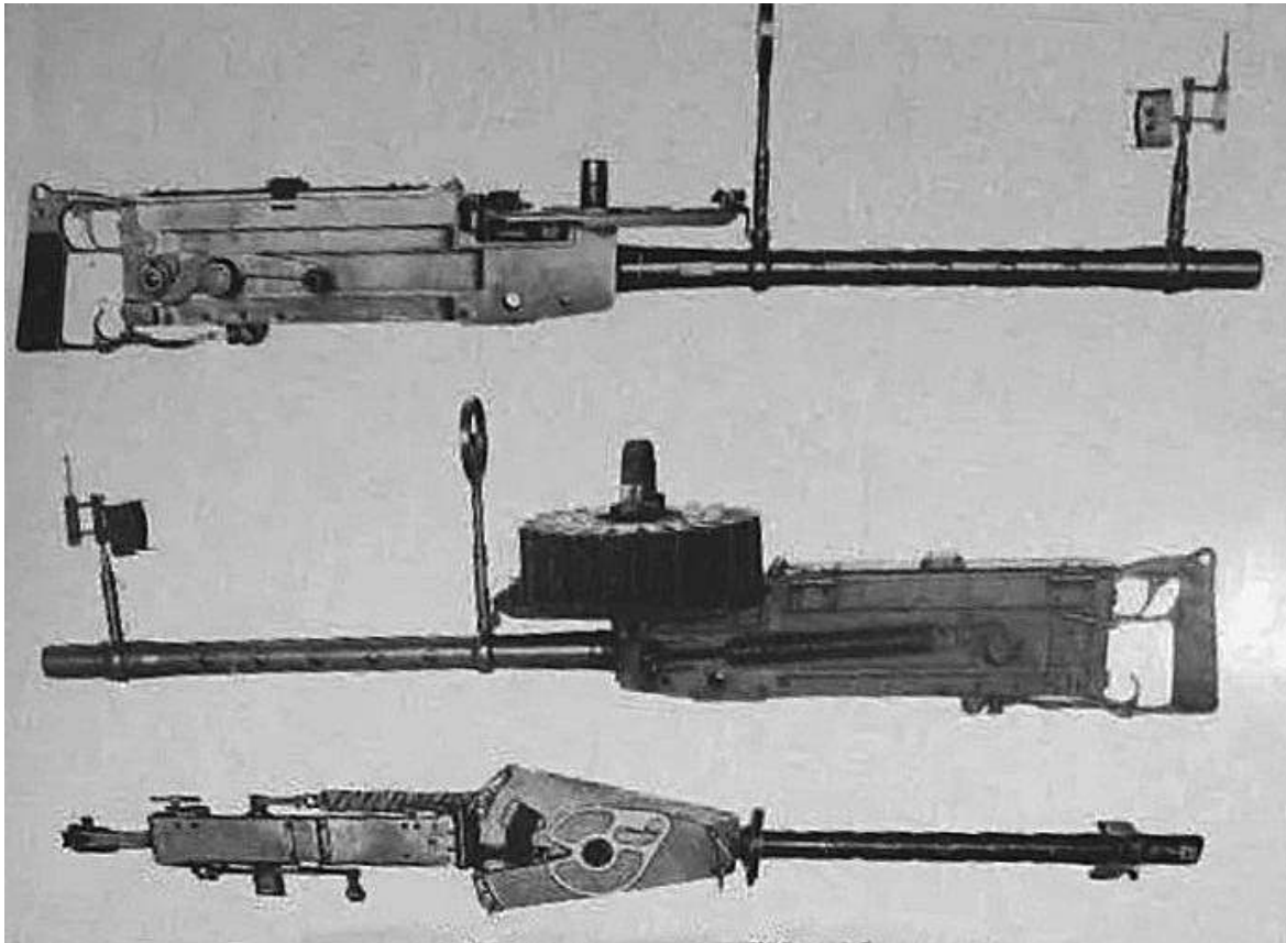
Ametralladora Vickers Mark "F".
