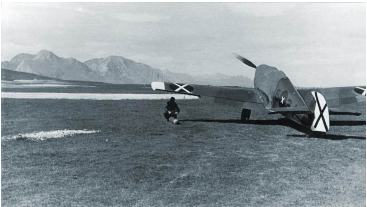
Los Messerschmitt Bf.109 B1 6-24 y 6-34 (página siguiente) en el aeródromo de Cué. Los monomotores de la Cónдор comenzaron a operar desde dicho aeródromo a poco de ser ocupado por las tropas nacionales. (Fotos colección de Eduardo Peralta).
