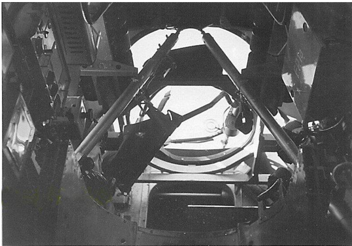
Puesto de ametralladora dorsal de un Heinkel He.111 fotografiado desde el interior del aparato. A la derecha del anillo puede adivinarse –más que verse– la Mg.15, con su cargador de doble tambor.
