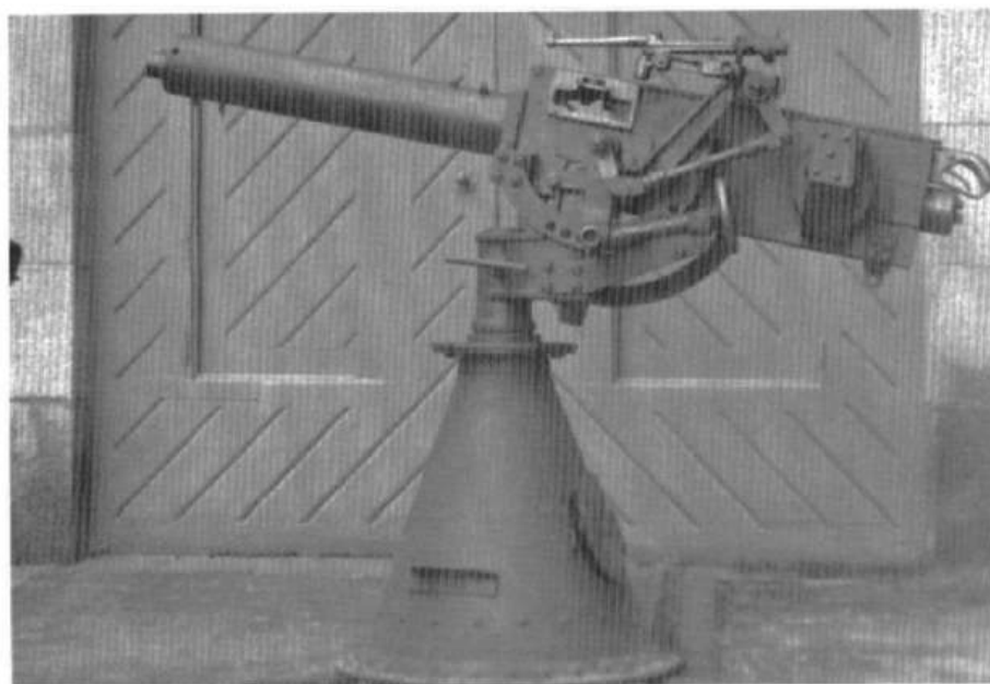
Ametralladora Maxim de 37 mm. transformada en antiaéreo de circunstancias en el Arsenal de Ferrol, para su propia defensa contra los bombardeos aéreos.
