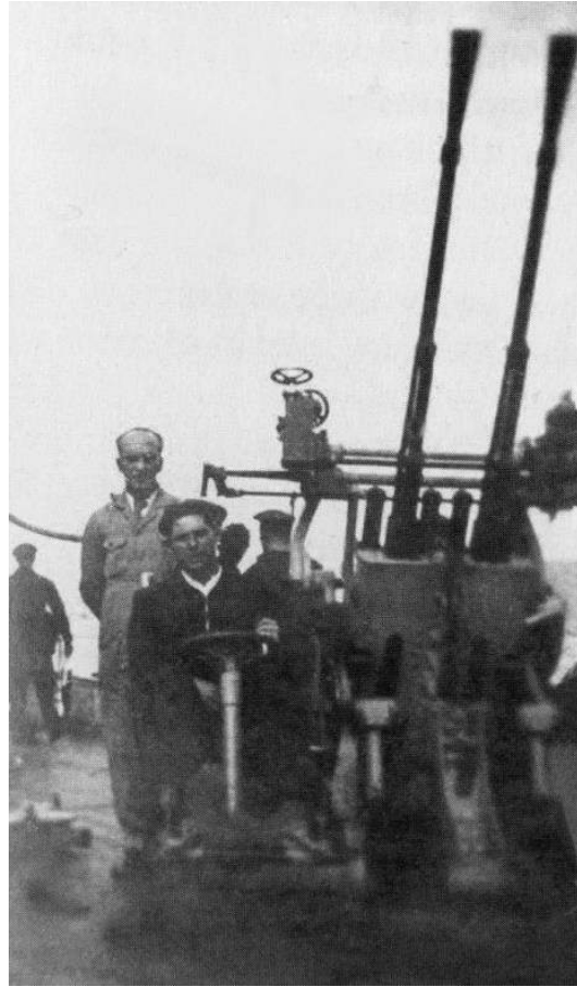
Izquierda. El Vickers de 76,2 mm. Mk. F.F. que montaba el "Císcar" era más antiguo y de peores características que el Mk. S,S, del "Díez" y de los demás destructores de su serie. Derecha. Montaje a/a. doble Hotchkiss de 25 mm del "José Luis Díez".
