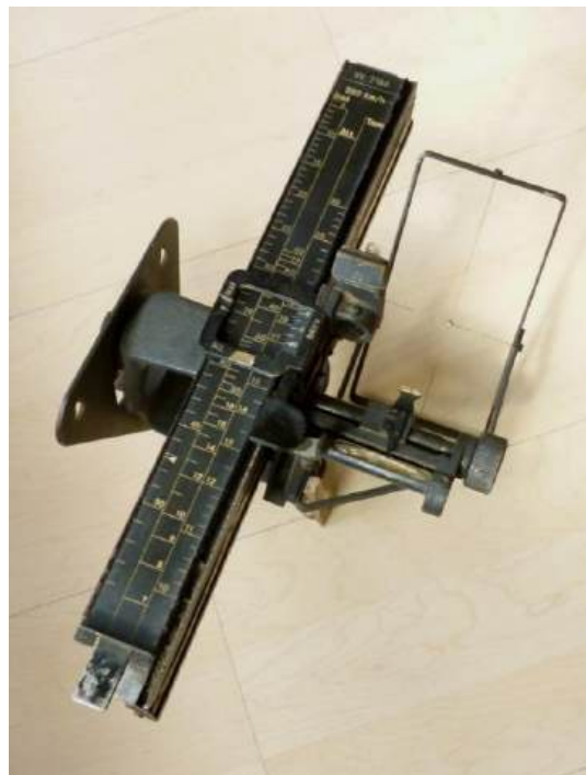
Visor Goerz Vizie 6V.219d empleado en los Ju.52 y por la mayor parte de los bombarderos suministrados por Alemania en los principios de su actuación en España (Museo Etnográfico y de Historia de Grado. Colección Guerra Civil en Asturias)
