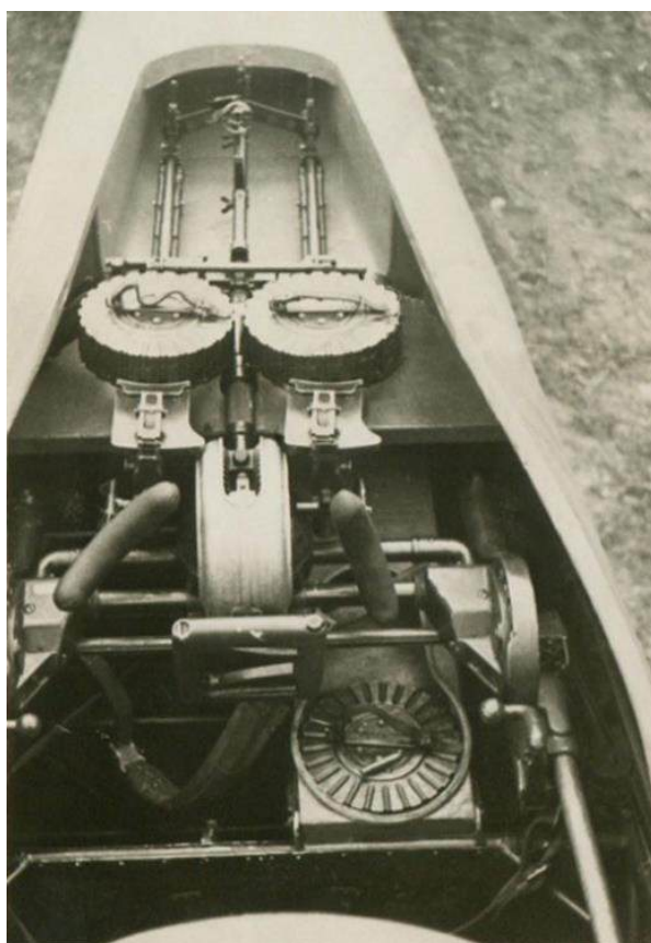
Montaje de metraladoras Lewis en el puesto del observador/bombardero. La imagen nos lo muestra en posición replegada, en la que no sobresalía del dorso del fuselaje
