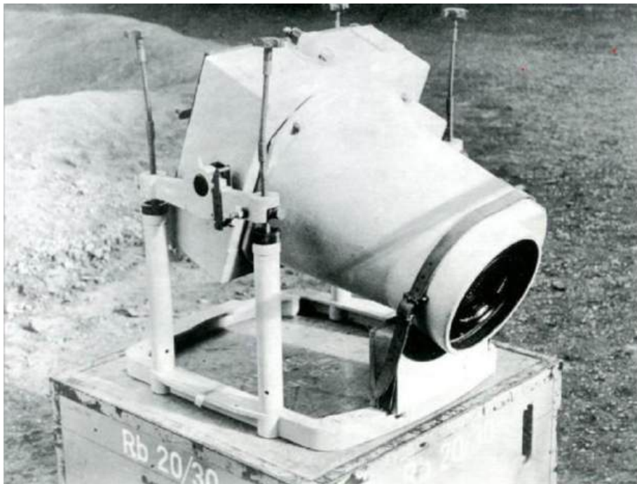
Cámara vertical Zeiss Rb 20/30, que utilizarían los Do.17 ya en 1938, en relevo de las Rb 10/18 o Rb21/18, de modelo más anticuado, con las que operaron en la campaña de Asturias.
