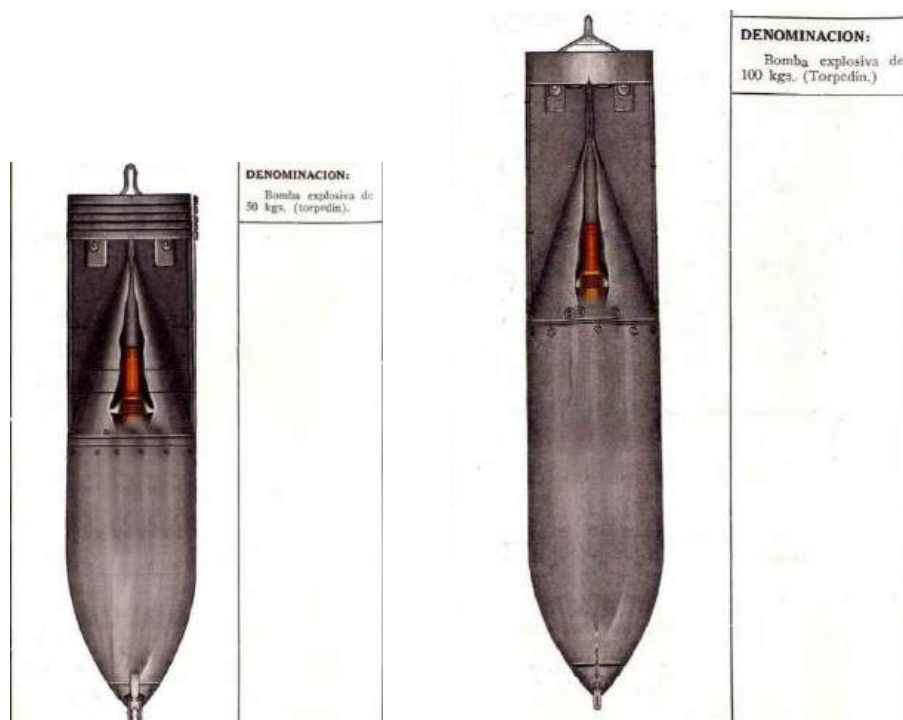
Bombas italianas Torpedini de 50 kg (izda.) y 100 kg (dcha.)
