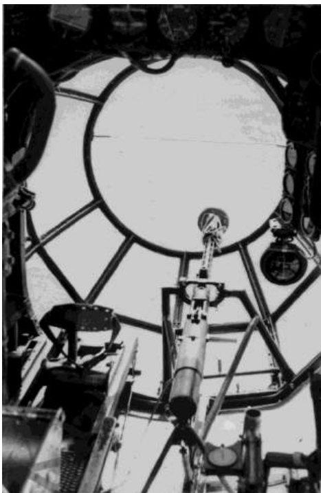
Sistema de engarce de la ametralladora MG.15 al afuste semi-rígido de proa.
