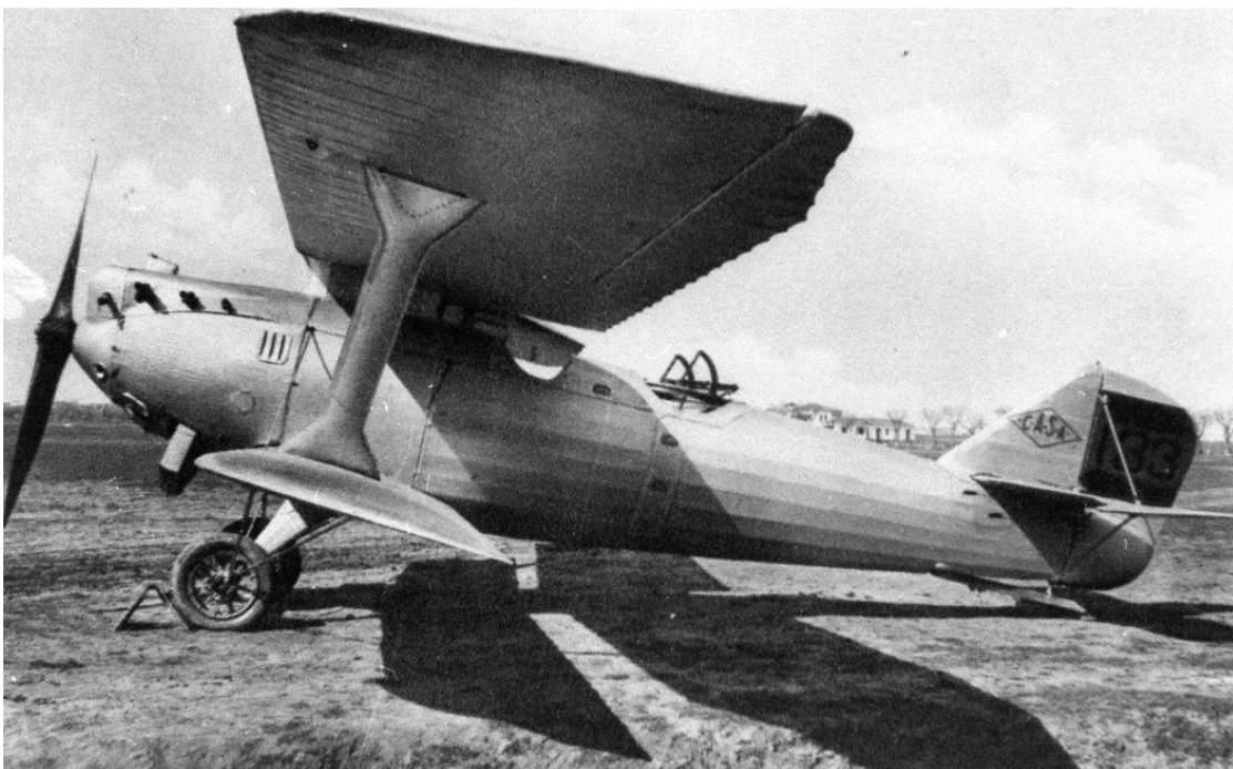
CASA/Breguet XIX con motor Hispano Suiza de 500 cv. Se trata del número de fabricación 133, último de la segunda serie española
