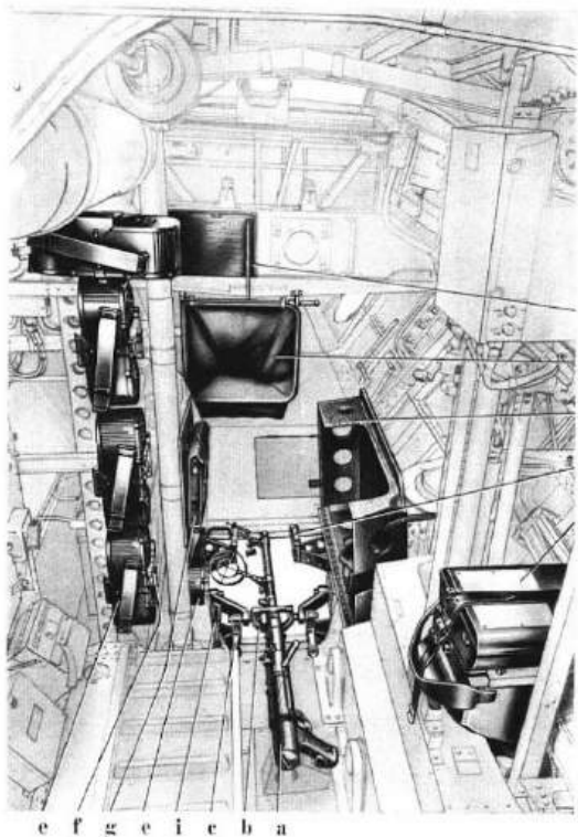
Puesto de ametralladora ventral de un Do.17. A la izquierda, abierto, listo para manejar el arma. A la derecha, aspecto del mismo puesto cerrado.
