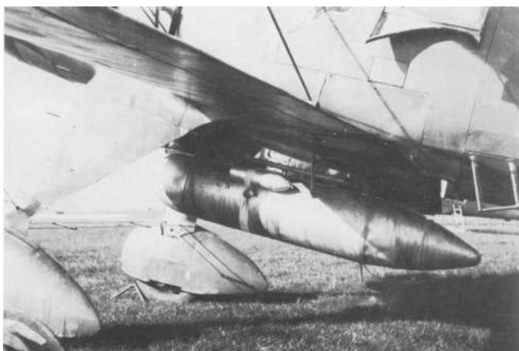
Depósito de combustible suplementario lanzable de un He.51 al que se ha sujetado con una cinta una pequeña bomba explosiva para transformarlo en el “temible” lanzallamas aéreo. En definitiva, una chapuza para tratar de prolongar la vida operativa del He.51.
