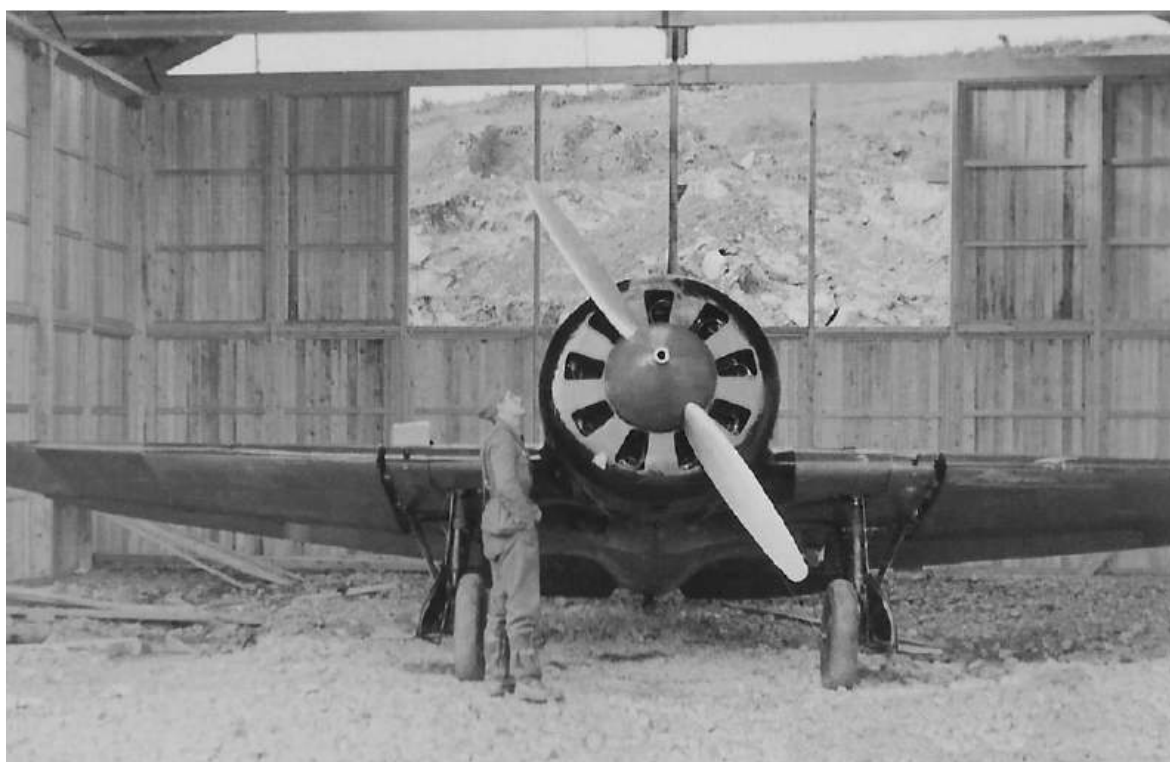
Polikarpov I.16 nº 33. El de mejor estado de entre los abandonados en Carreño. Tan bueno –casi en condiciones de vuelo.(El único daño que se aprecia es la rotura del extremo posterior del puro que dejó sin soporte al patín de cola, por lo que fue necesario utilizar para moverlo el carrito de dos ruedas que se ve tras él)- los miembros de la Cónдор se apresuraron a “requisarlo” y enviarlo a Alemania. (Foto Otto Schmidt, cedida por su hijo Heli Schmidt)
