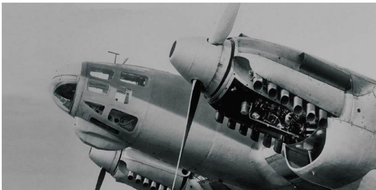
Motores DB 600 Aa de un He.111 B-0.
