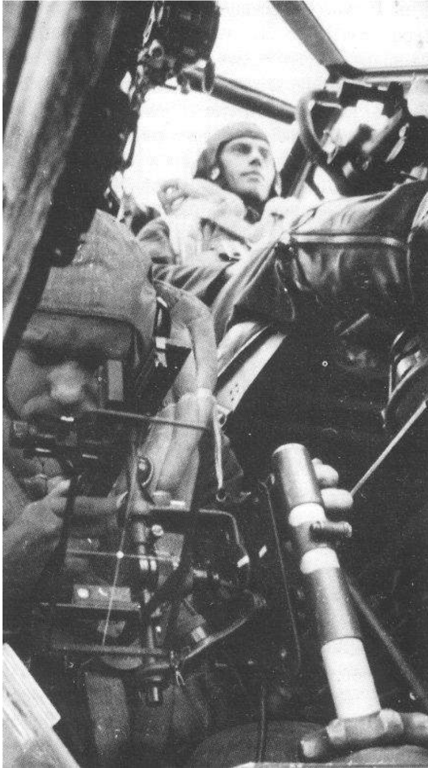
El observador-bombardero de un Do.17 ajusta la puntería de su visor Goerz 6V.219d para localizar el objetivo, presumiblemente próximo.
