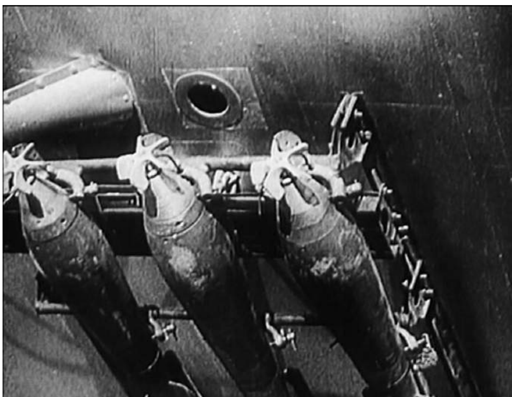
Fotografía de detalle de un lanzabombas 3-A-5, con tres Hispania A.5 –de 12 kg.-, montado en un Breguet XIX.
