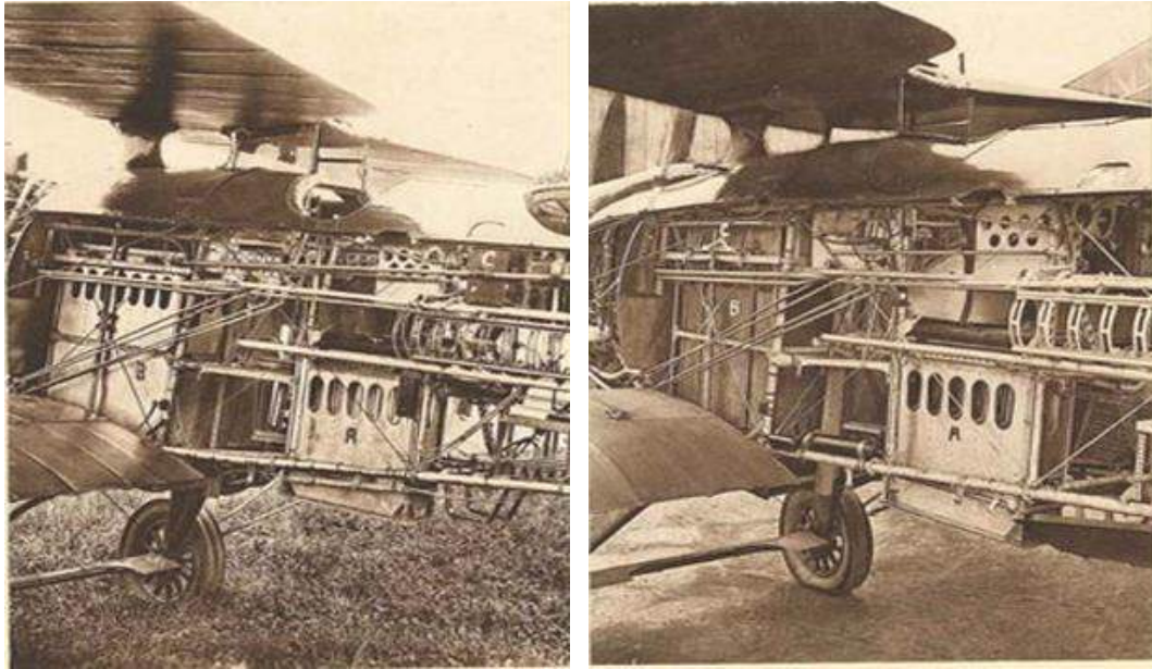
(Izda.) Breguet XIX B 2, de bombardeo, mostrando los lanzabombas pequeño, para 12 bombas de 10/14 kg (A) y grande para 32 bombas de 12/14 kg o para 8 con un peso unitario de 50/54 (B). (Dcha.) Breguet XIX A2, de reconocimiento; se aprecia el lanzabombas pequeño (A) y el compartimento para la cámara fotográfica (B) en sustitución del lanzabombas grande.
