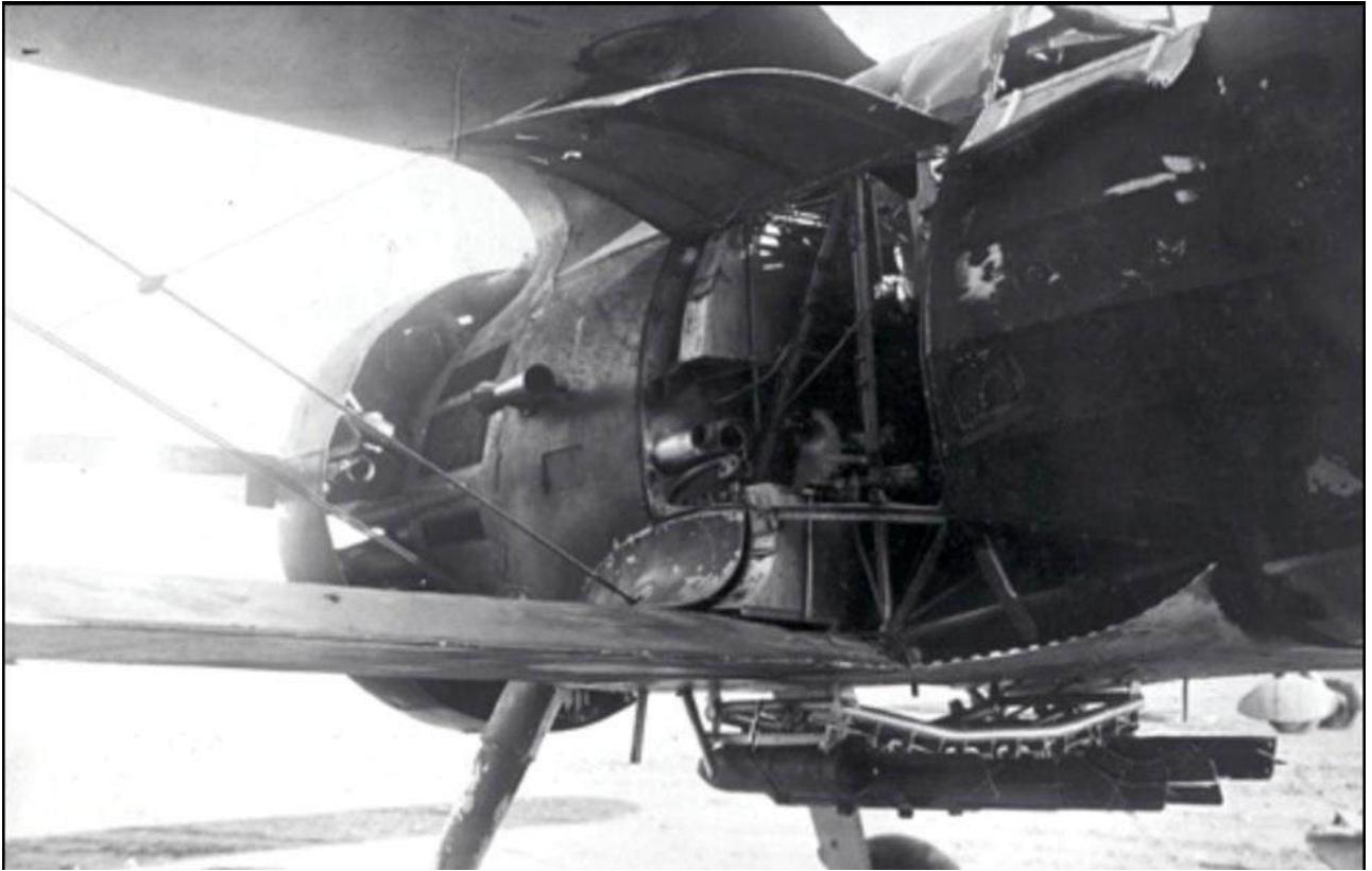
Polikarpov I.15 equipado con el lanzabombas para 8 bombas de 10 kilos.
