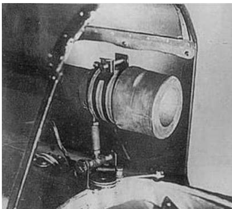
Detalle del mismo visor OP-1, mostrando el apoyo de caucho para la frente del piloto.
