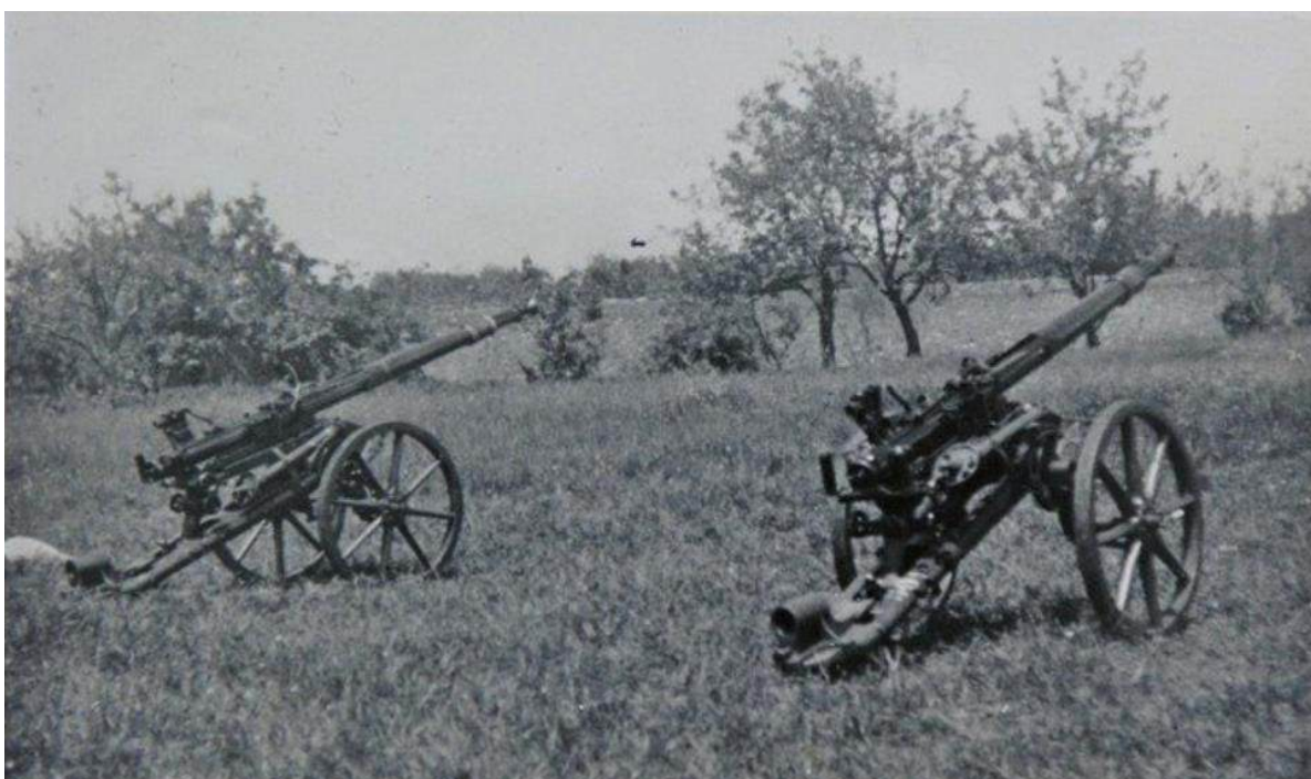
Ametralladoras Semag de 20 mm Tipo L en configuración de tiro terrestre.
