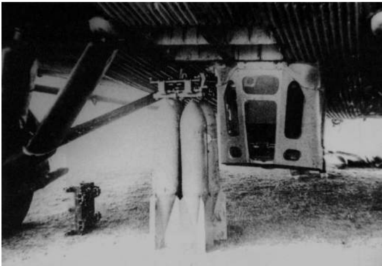
Cuatro bombas SC/50 dispuestas para ser izadas al pozo delantero de un Ju.52. Se hallan enganchadas al cuadrante que permite acoplarlas y manejarlas desde un lanzabombas diseñado para una sola de 250 kg. En ambas fotos se aprecia en el suelo, suelto, uno de tales cuadrantes.
