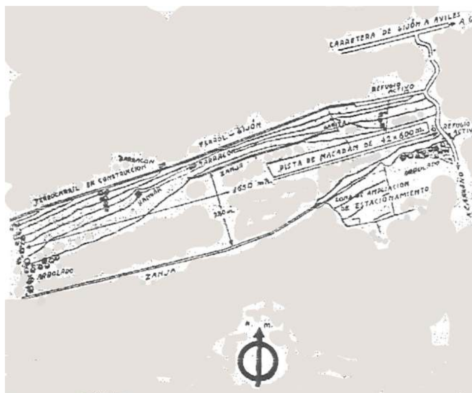
Plano del aeródromo de Carreño.
