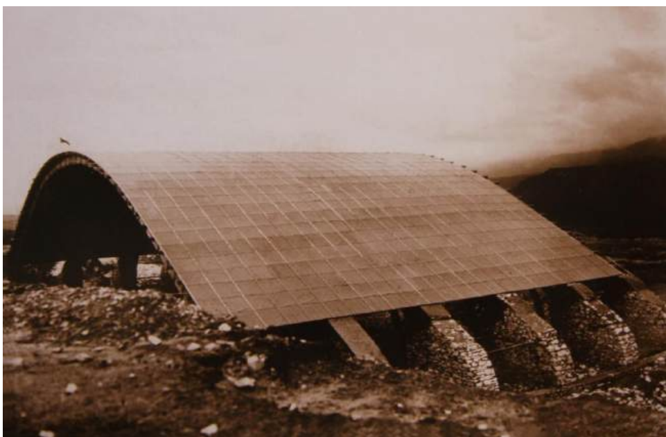
El curioso hangar del aeródromo de Cué en estado de avanzada construcción.
