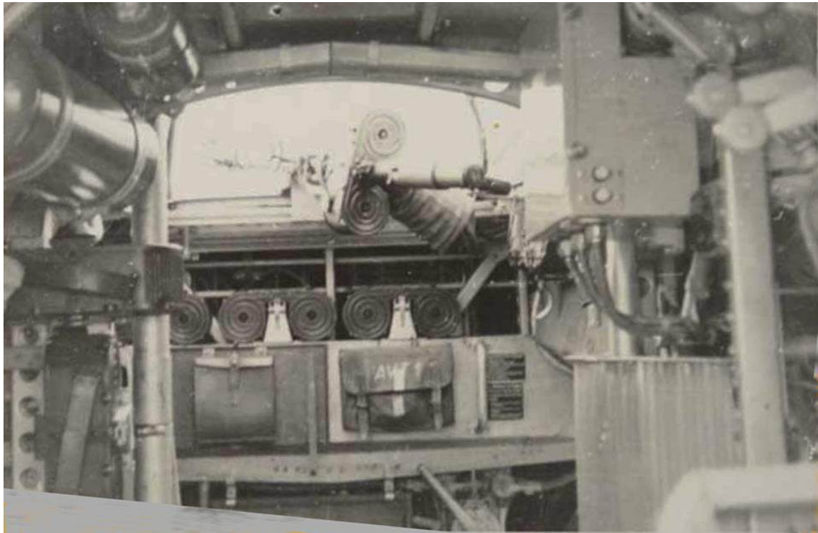
Vista desde el interior del puesto de ametralladora dorsal en una imagen que nos permite apreciar nuevos detalles.
